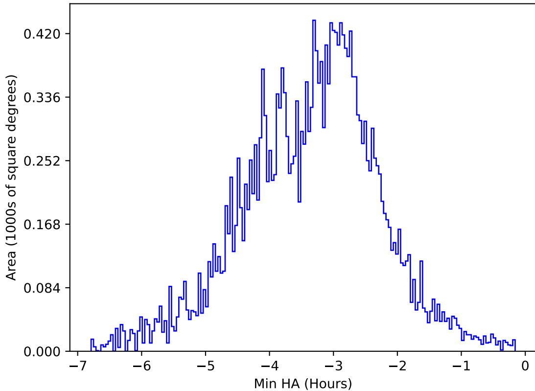
mw_roll_all_v3.3_10yrs All sky y band: Min HA
