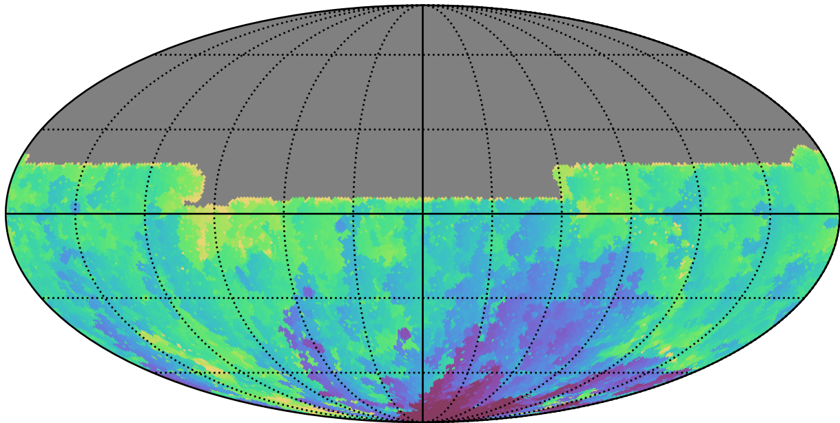
mw_roll_all_v3.3_10yrs All sky u band: Min HA
