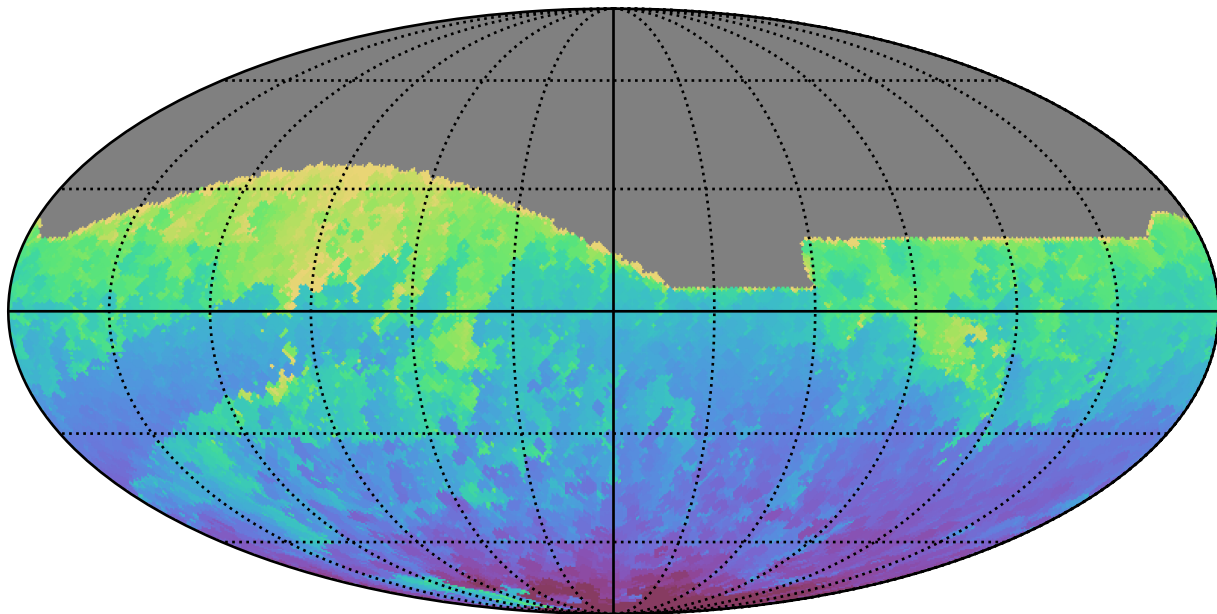
mw_roll_all_v3.3_10yrs All sky i band: Min HA
