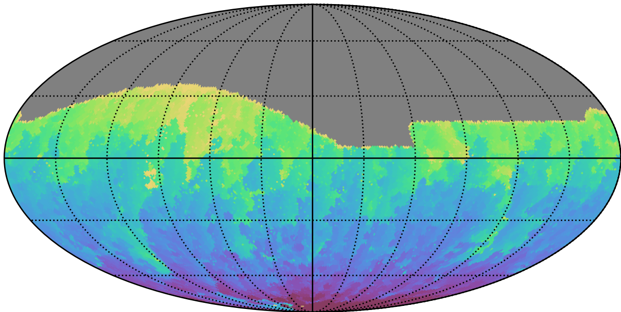
mw_roll_all_v3.3_10yrs All sky g band: Min HA
