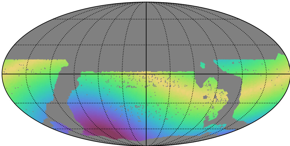
mw_roll_all_v3.3_10yrs WFD y band: Max solarElong
