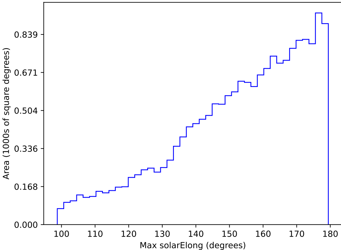
mw_roll_all_v3.3_10yrs WFD y band: Max solarElong
