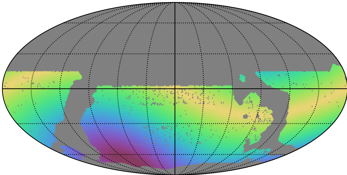
mw_roll_all_v3.3_10yrs WFD i band: Max solarElong
