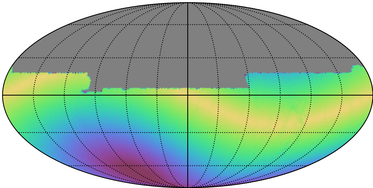
mw_roll_all_v3.3_10yrs All sky y band: Max solarElong
