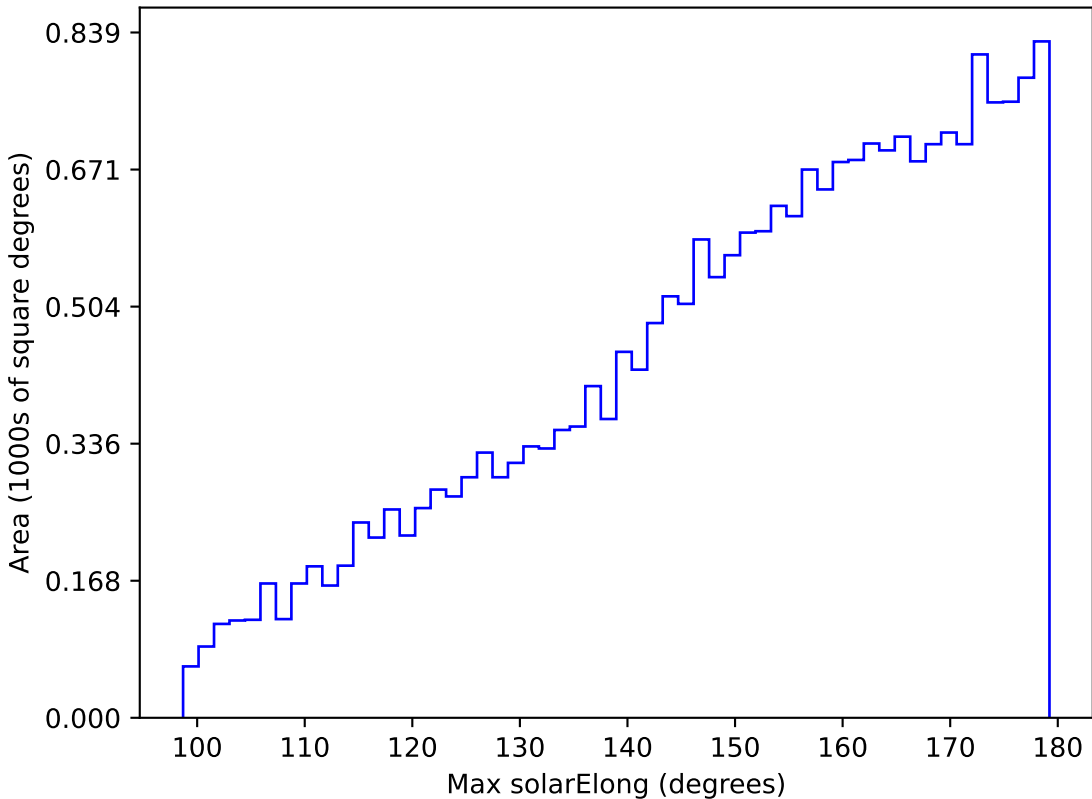
mw_roll_all_v3.3_10yrs All sky y band: Max solarElong
