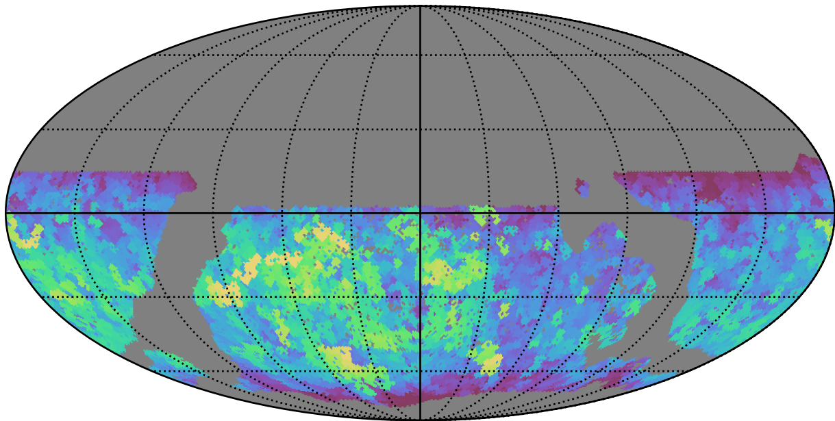
mw_roll_all_v3.3_10yrs WFD z band: Max saturation_mag
