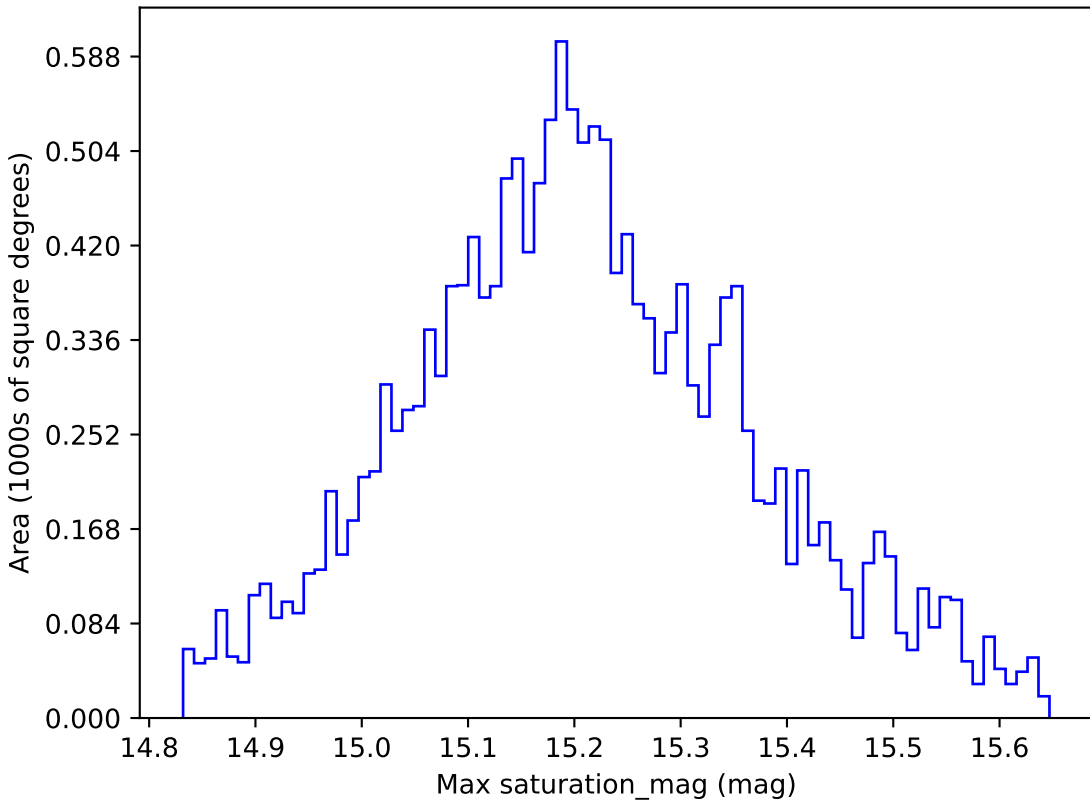
mw_roll_all_v3.3_10yrs WFD z band: Max saturation_mag
