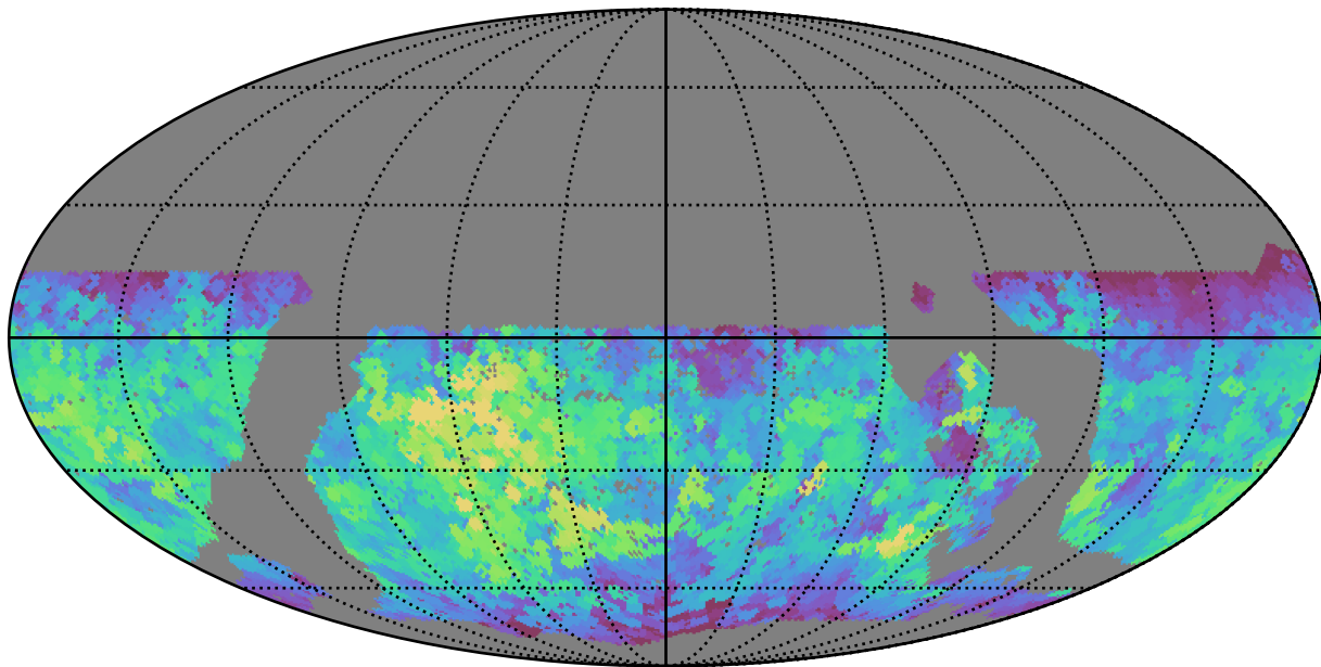
mw_roll_all_v3.3_10yrs WFD y band: Max saturation_mag
