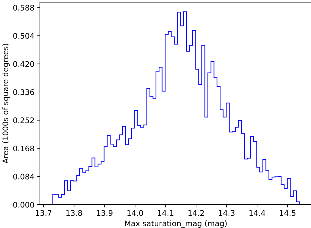
mw_roll_all_v3.3_10yrs WFD y band: Max saturation_mag
