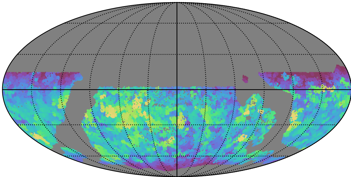
mw_roll_all_v3.3_10yrs WFD r band: Max saturation_mag
