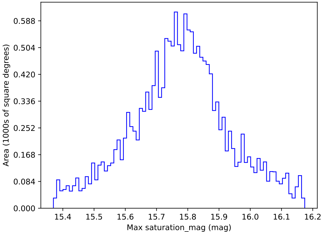
mw_roll_all_v3.3_10yrs WFD r band: Max saturation_mag
