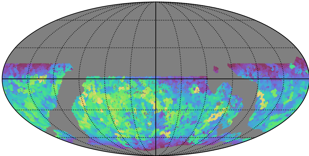
mw_roll_all_v3.3_10yrs WFD i band: Max saturation_mag
