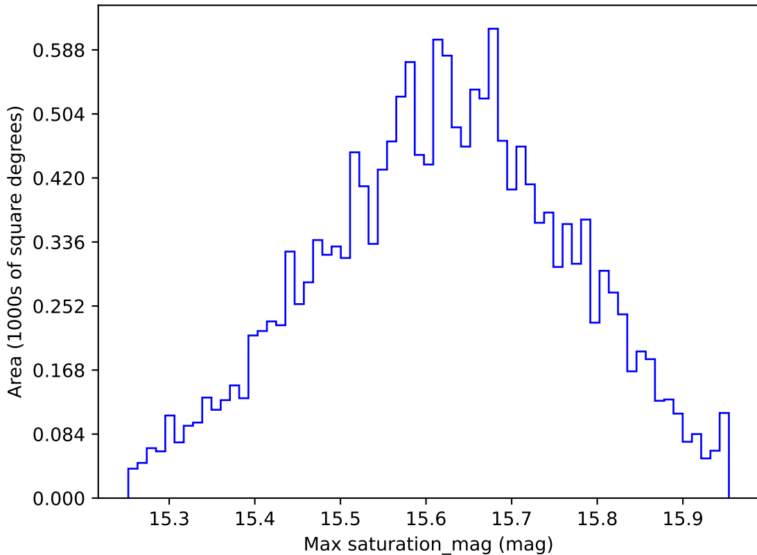
mw_roll_all_v3.3_10yrs WFD i band: Max saturation_mag
