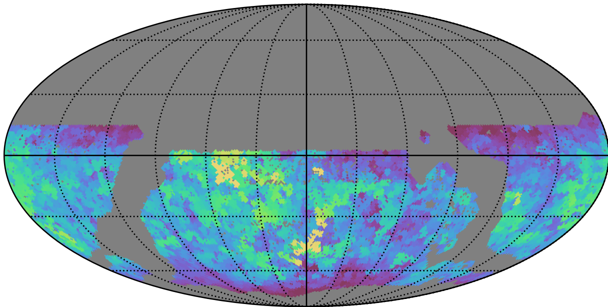
mw_roll_all_v3.3_10yrs WFD g band: Max saturation_mag
