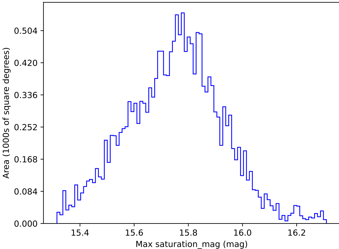
mw_roll_all_v3.3_10yrs WFD g band: Max saturation_mag
