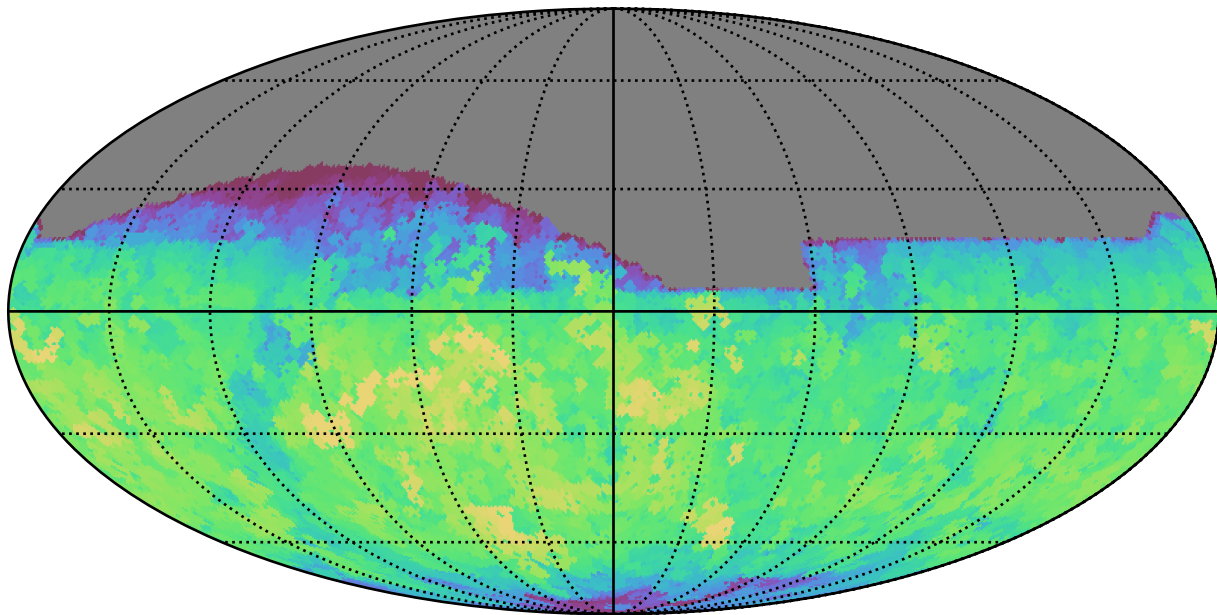
mw_roll_all_v3.3_10yrs All sky z band: Max saturation_mag
