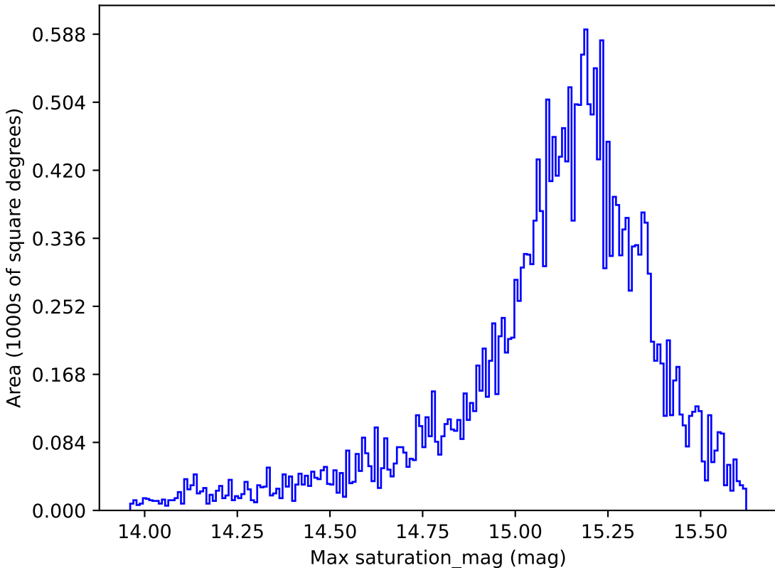
mw_roll_all_v3.3_10yrs All sky z band: Max saturation_mag
