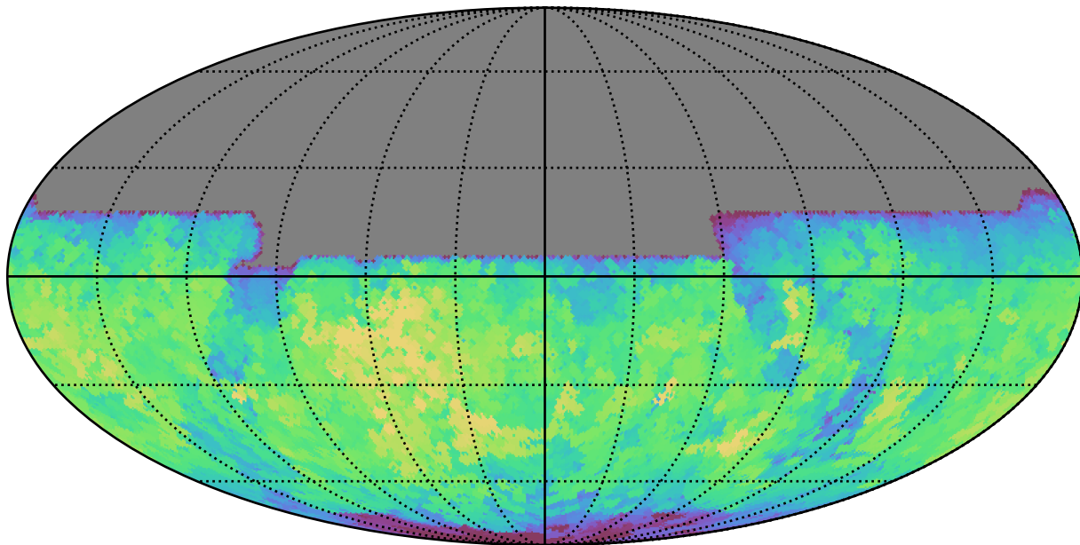
mw_roll_all_v3.3_10yrs All sky y band: Max saturation_mag
