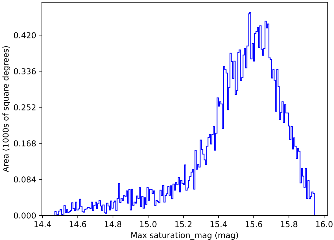
mw_roll_all_v3.3_10yrs All sky i band: Max saturation_mag
