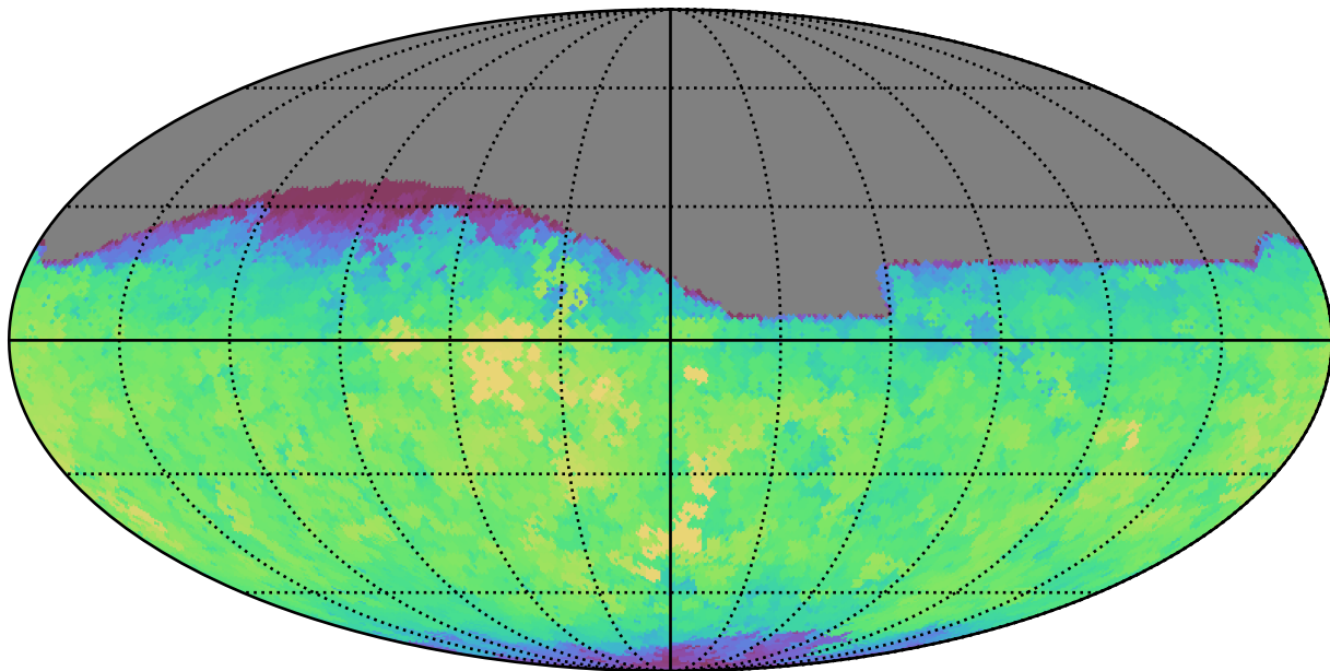
mw_roll_all_v3.3_10yrs All sky g band: Max saturation_mag
