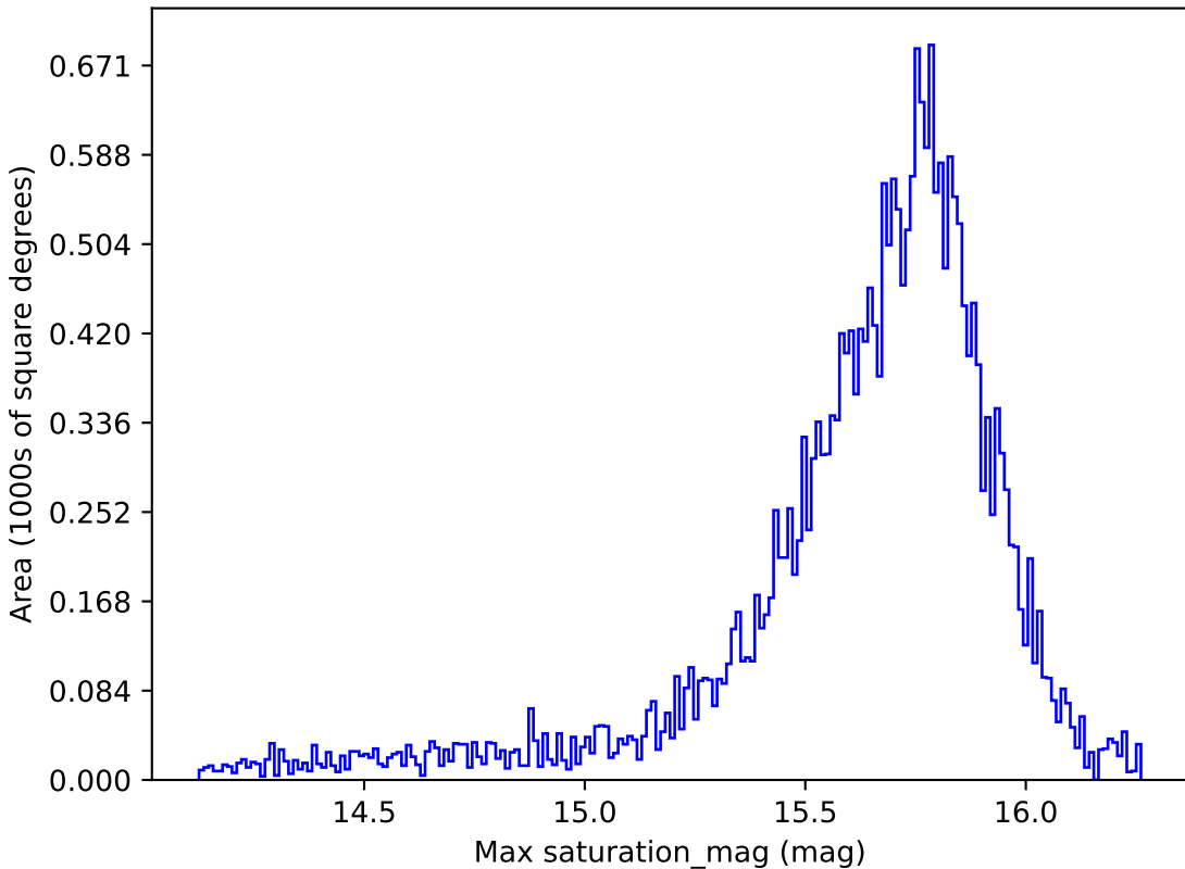
mw_roll_all_v3.3_10yrs All sky g band: Max saturation_mag
