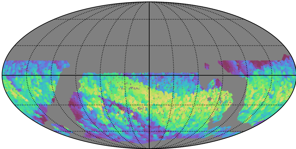
mw_roll_all_v3.3_10yrs WFD z band: Max normairmass
