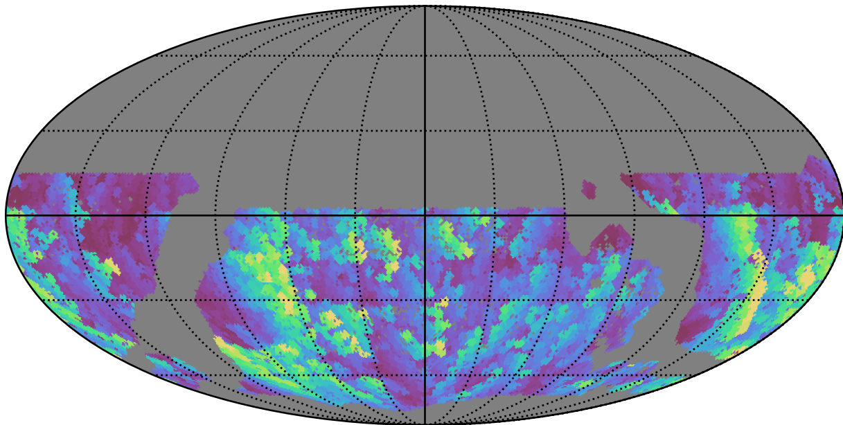
mw_roll_all_v3.3_10yrs WFD u band: Max normairmass
