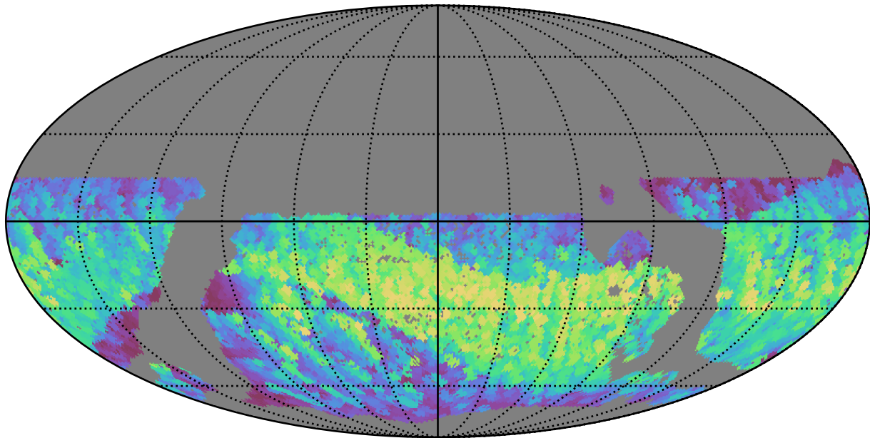
mw_roll_all_v3.3_10yrs WFD i band: Max normairmass
