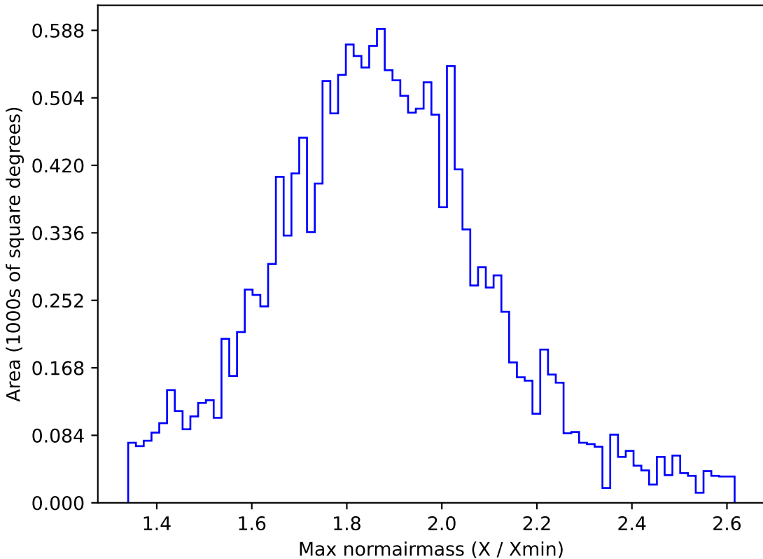
mw_roll_all_v3.3_10yrs WFD g band: Max normairmass
