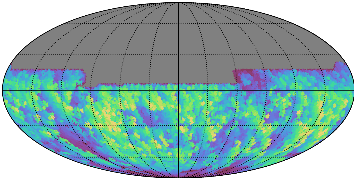
mw_roll_all_v3.3_10yrs All sky y band: Max normairmass
