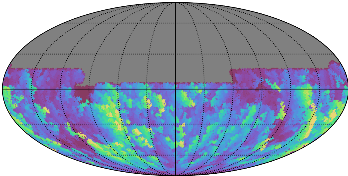
mw_roll_all_v3.3_10yrs All sky u band: Max normairmass
