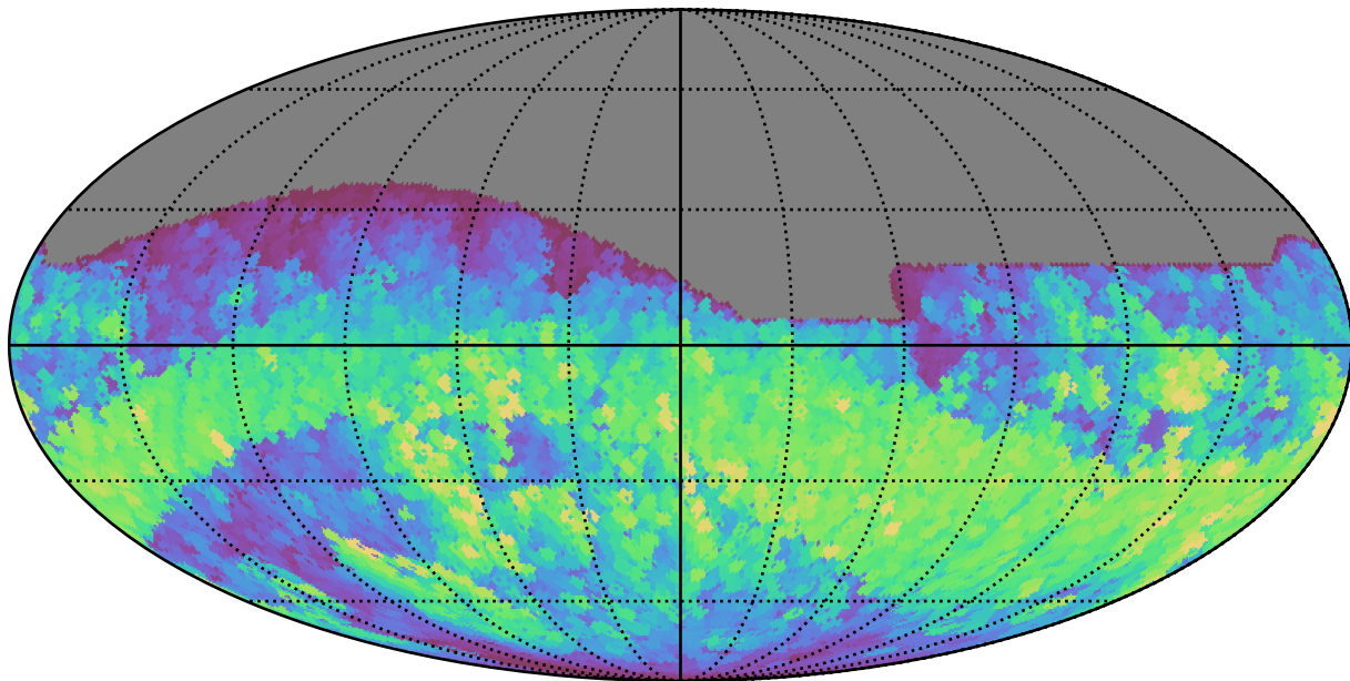
mw_roll_all_v3.3_10yrs All sky r band: Max normairmass
