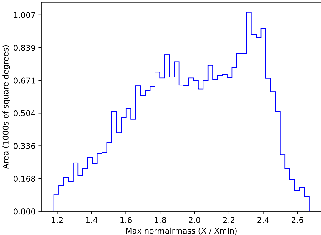
mw_roll_all_v3.3_10yrs All sky r band: Max normairmass
