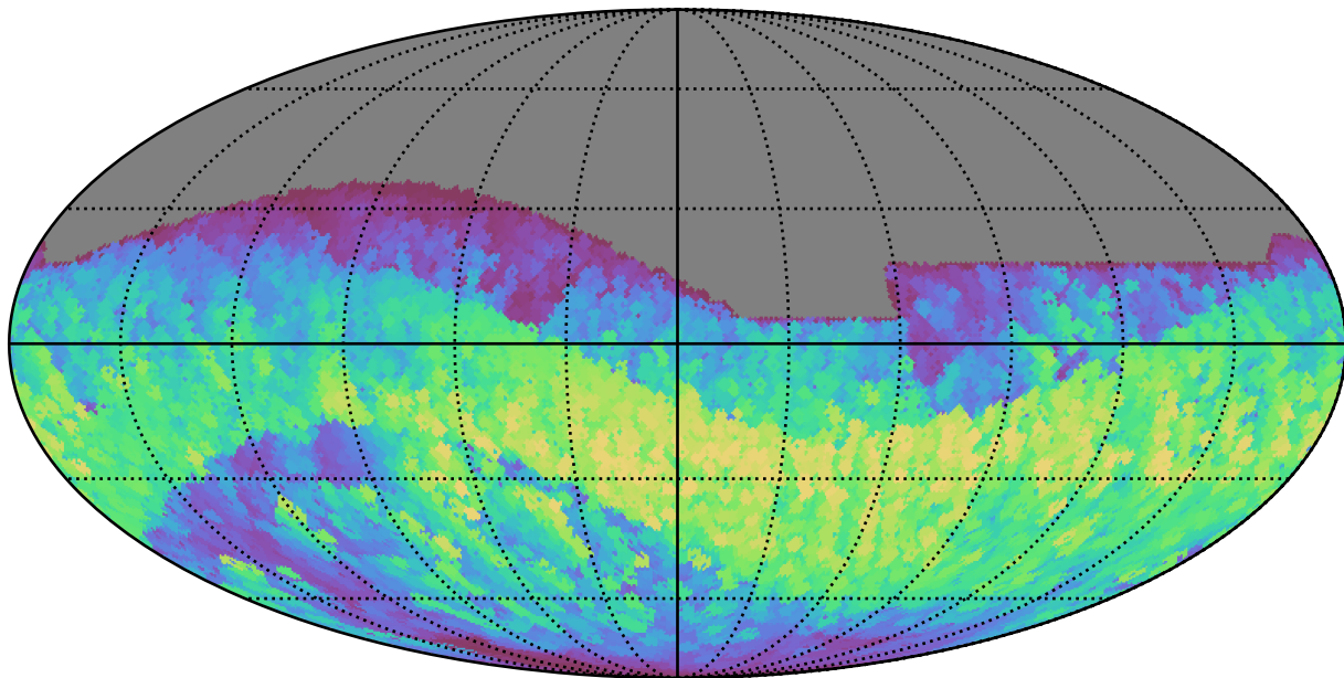
mw_roll_all_v3.3_10yrs All sky i band: Max normairmass
