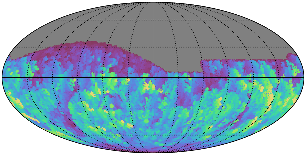
mw_roll_all_v3.3_10yrs All sky g band: Max normairmass
