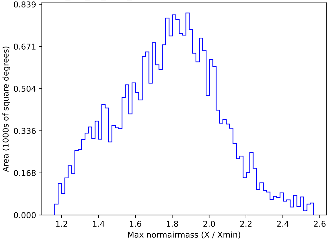
mw_roll_all_v3.3_10yrs All sky g band: Max normairmass
