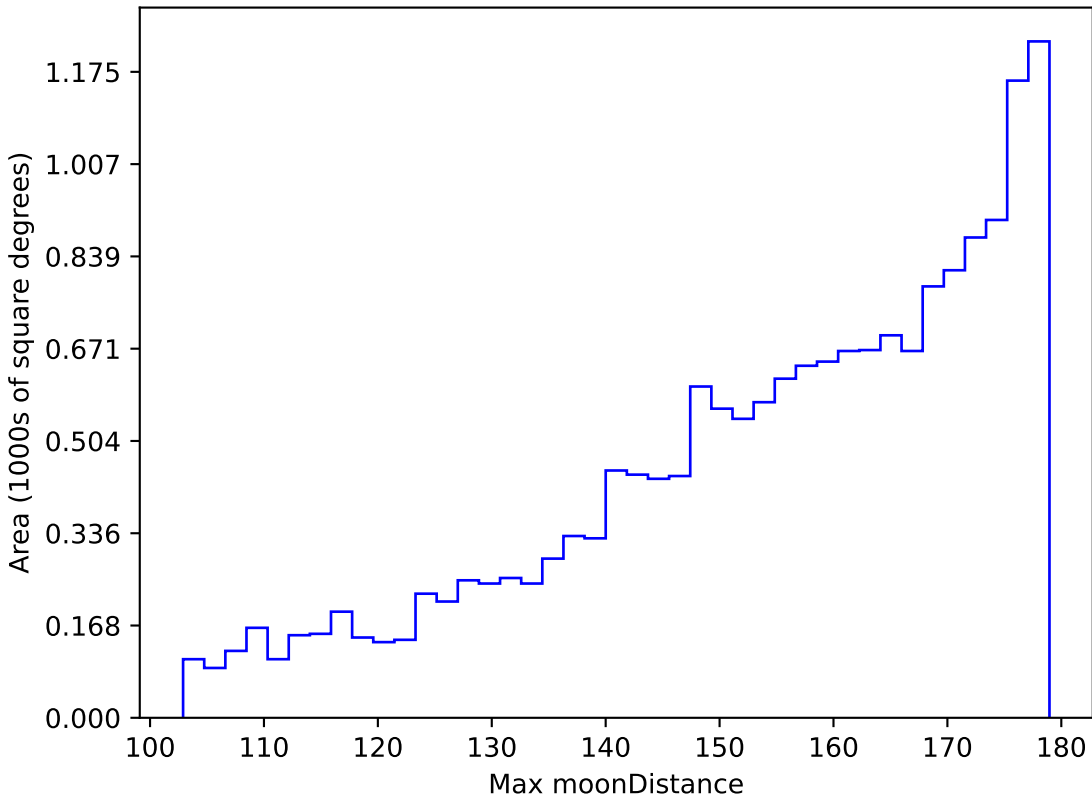
mw_roll_all_v3.3_10yrs WFD z band: Max moonDistance
