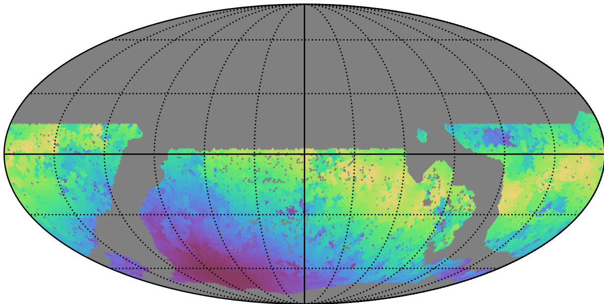
mw_roll_all_v3.3_10yrs WFD y band: Max moonDistance
