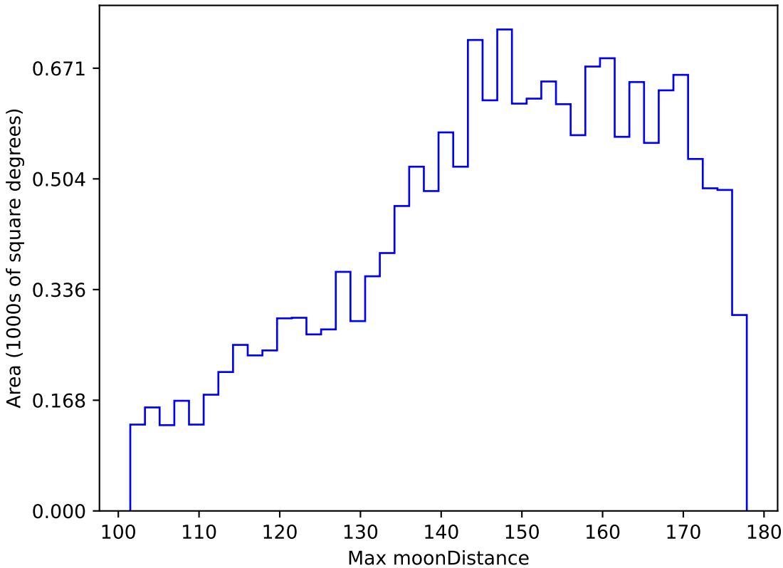
mw_roll_all_v3.3_10yrs WFD y band: Max moonDistance
