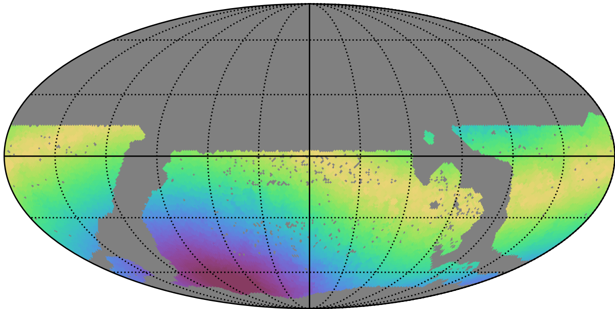
mw_roll_all_v3.3_10yrs WFD i band: Max moonDistance
