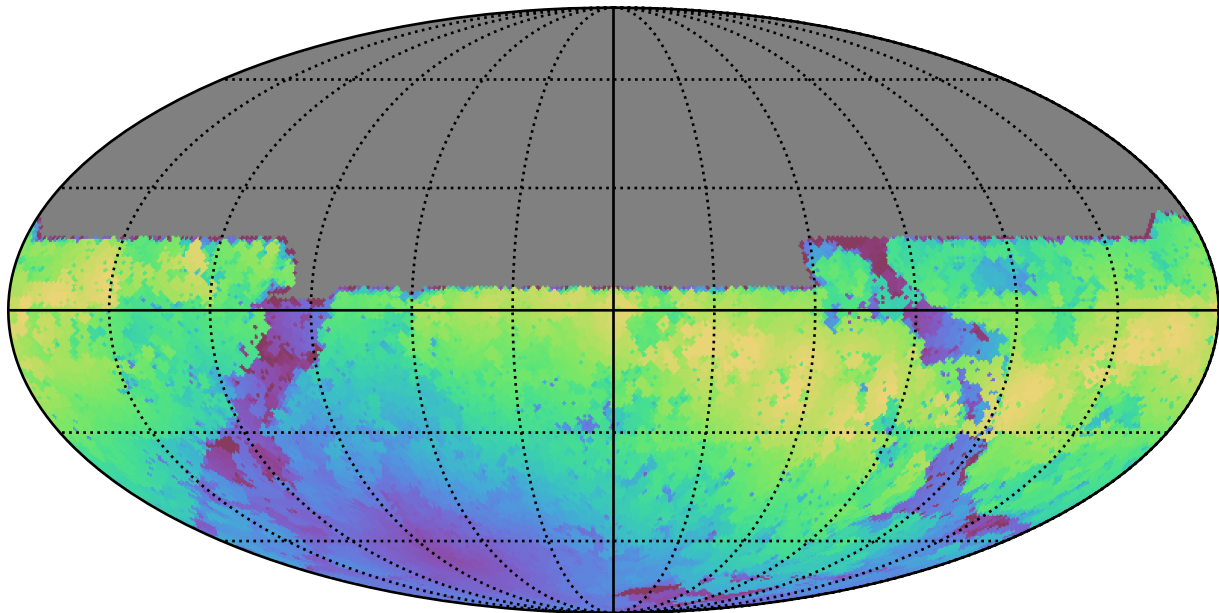
mw_roll_all_v3.3_10yrs All sky y band: Max moonDistance
