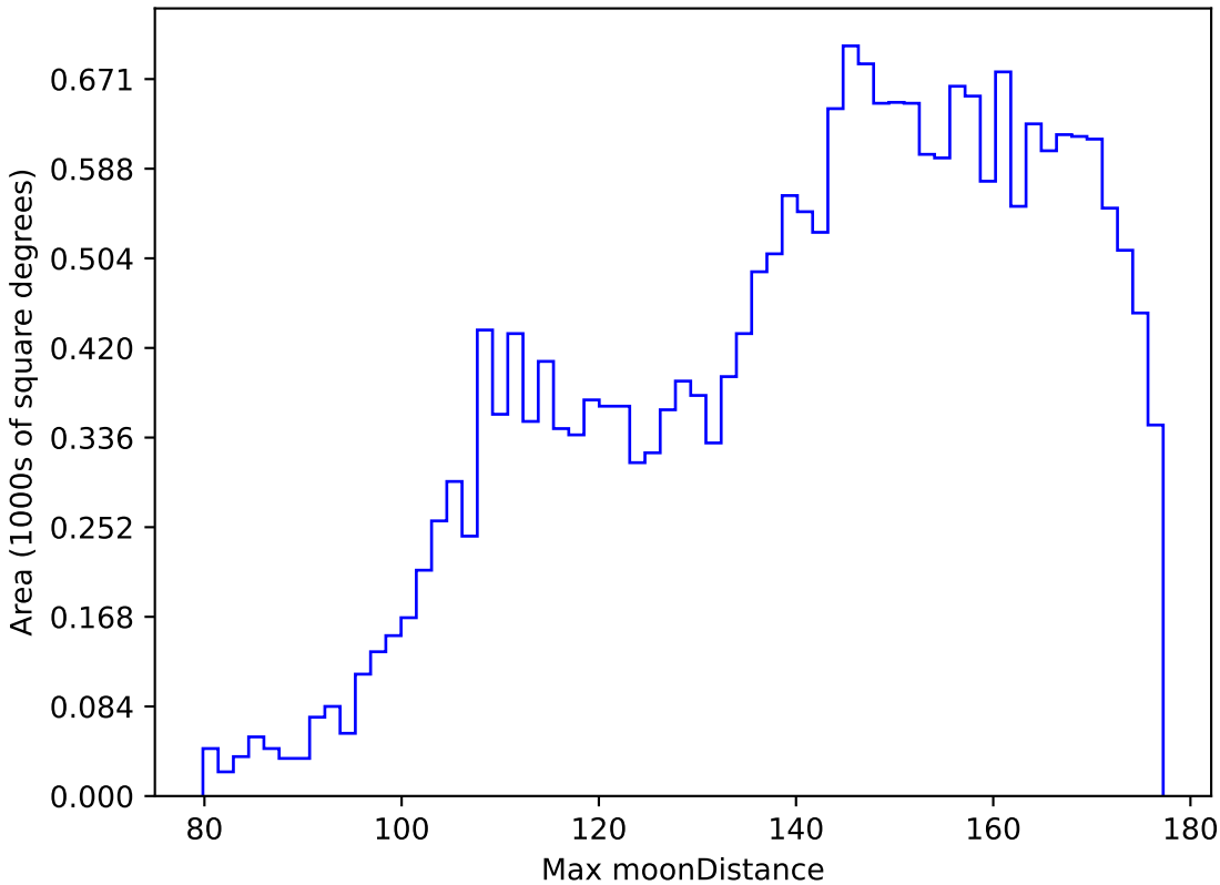
mw_roll_all_v3.3_10yrs All sky y band: Max moonDistance
