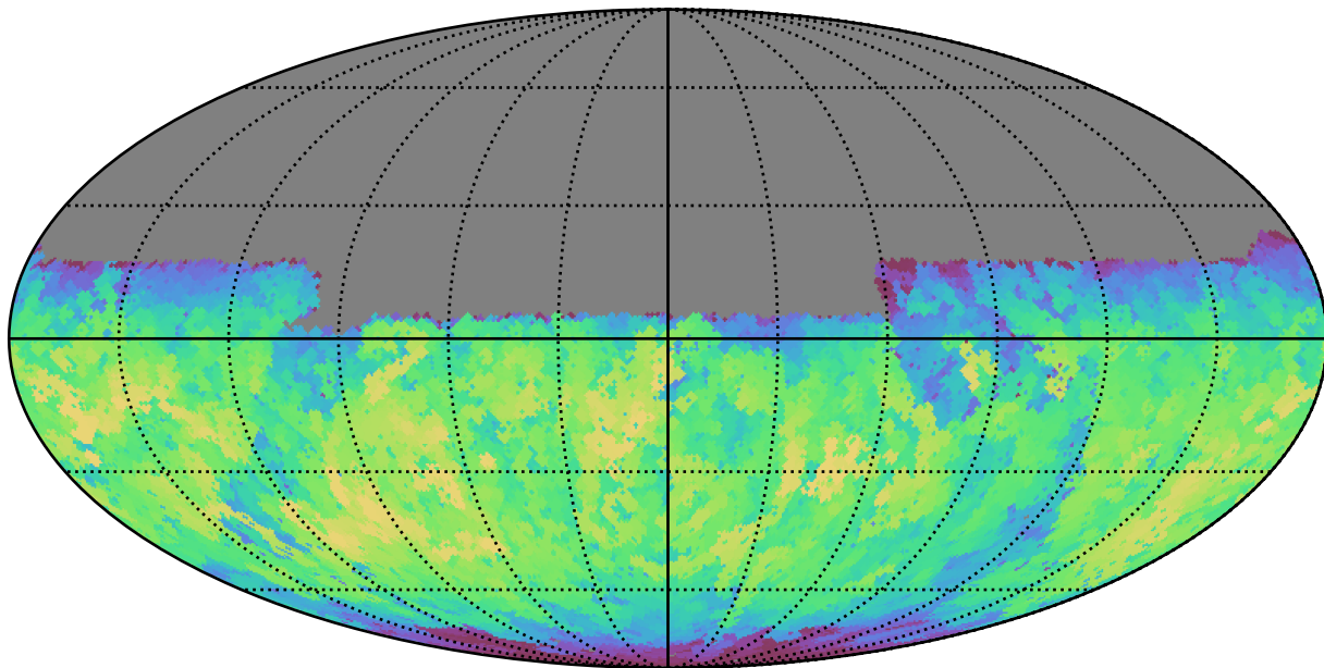
mw_roll_all_v3.3_10yrs Yr 1 y band: Max fiveSigmaDepth
