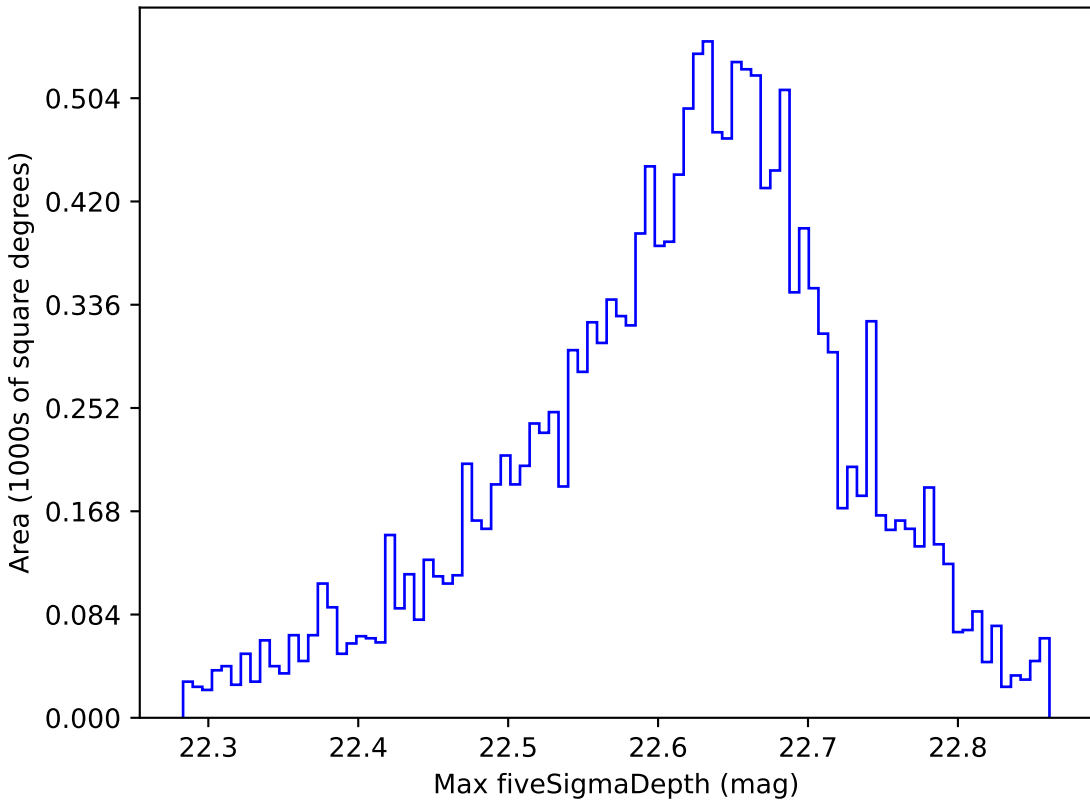
mw_roll_all_v3.3_10yrs WFD y band: Max fiveSigmaDepth
