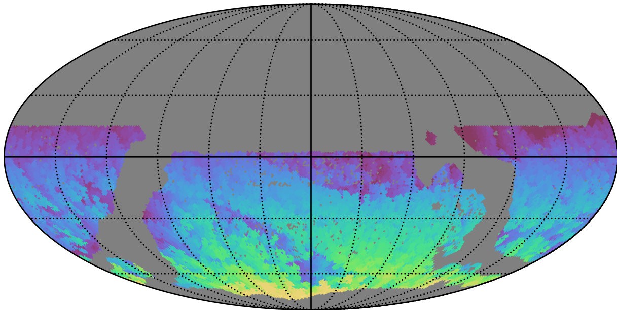
mw_roll_all_v3.3_10yrs WFD z band: Max HA
