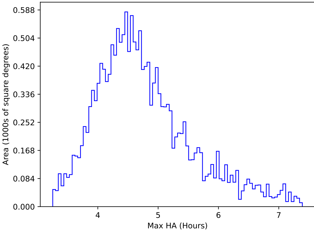
mw_roll_all_v3.3_10yrs WFD y band: Max HA
