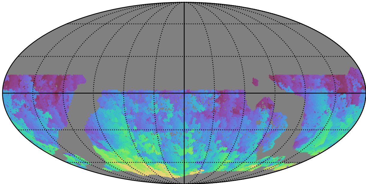
mw_roll_all_v3.3_10yrs WFD u band: Max HA
