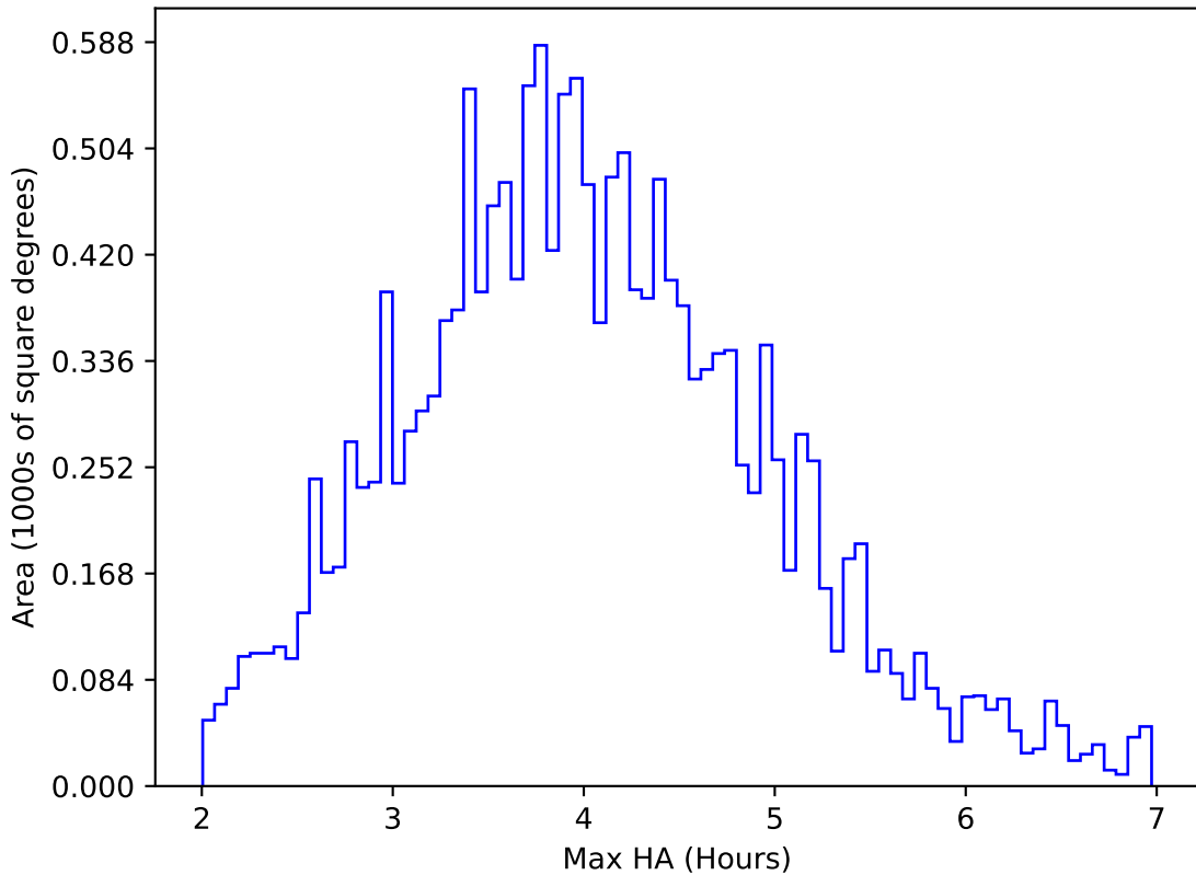
mw_roll_all_v3.3_10yrs WFD u band: Max HA
