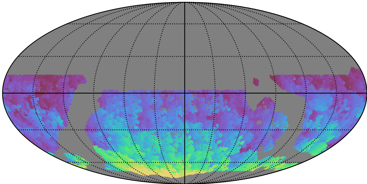
mw_roll_all_v3.3_10yrs WFD r band: Max HA
