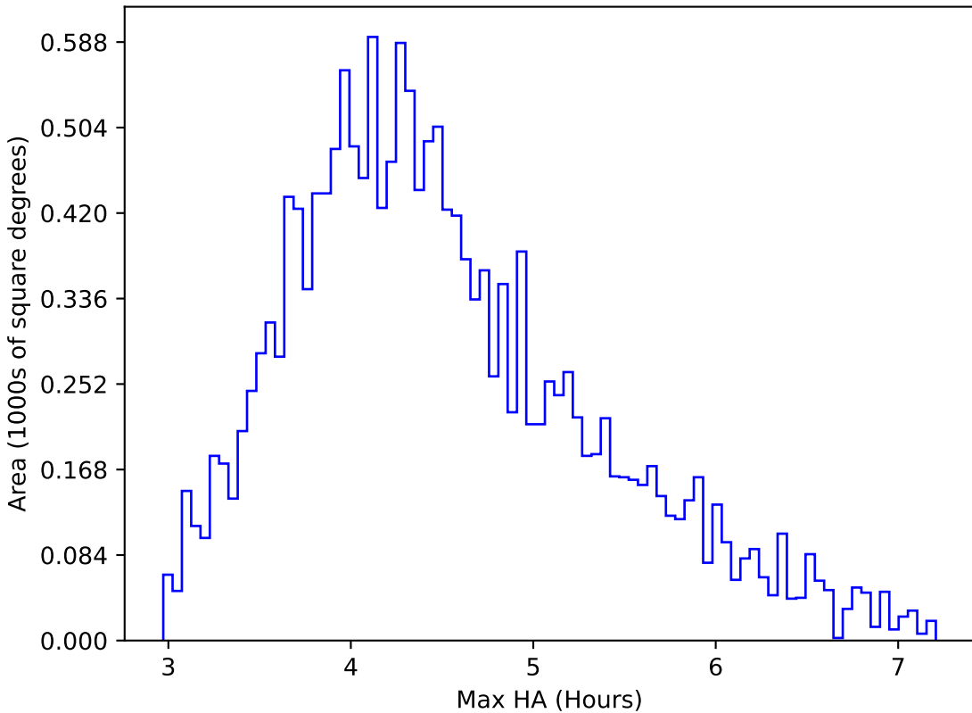
mw_roll_all_v3.3_10yrs WFD r band: Max HA
